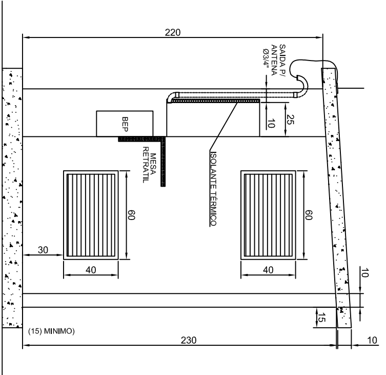
CORTE B-B'
